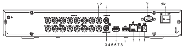
DH-XVR5216AN-4KL-X
